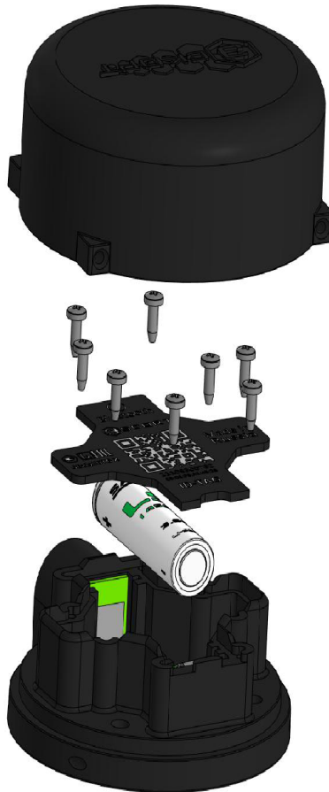
Рисунок 1 – Конструкция метки беспроводной «Escort TAG»
